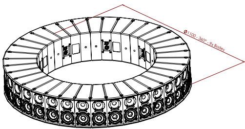
360° 配置模板 (尺寸单位: mm)
